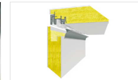
SEZIONE TETTO | CEILING SECTION ROOF
