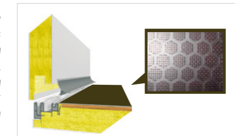
SEZIONE PAVIMENTO | FLOOR SECTION
