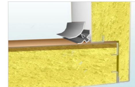
SEZIONE PAVIMENTO | FLOOR SECTION
